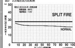
図2 2次電圧出力比較表
