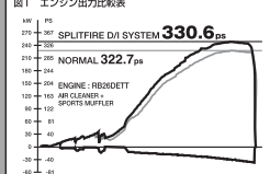
図1 エンジン出力比較表
